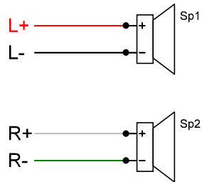
2 x 8 ohm Speakers 2 x 8 Ohm Lautsprecher
