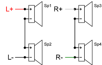
4 x 4 ohm Speakers 4 x 4 Ohm Lautsprecher
