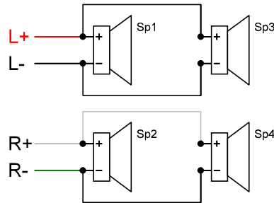
4 x 16 ohm Speakers 4 x 16 Ohm Lautsprecher
