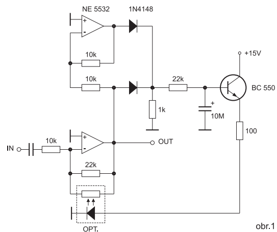
Princip zapojení limiteru s nízkým zkreslením Schematic circuit diagram of limiter with low distortion
